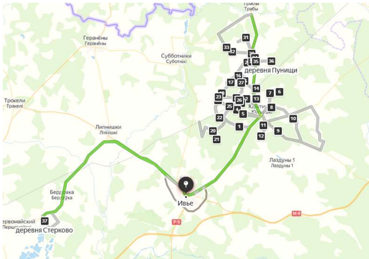
Рисунок 14 – Маршрутный график сбора и удаления ТКО машина 2 1й и 3й чт.
