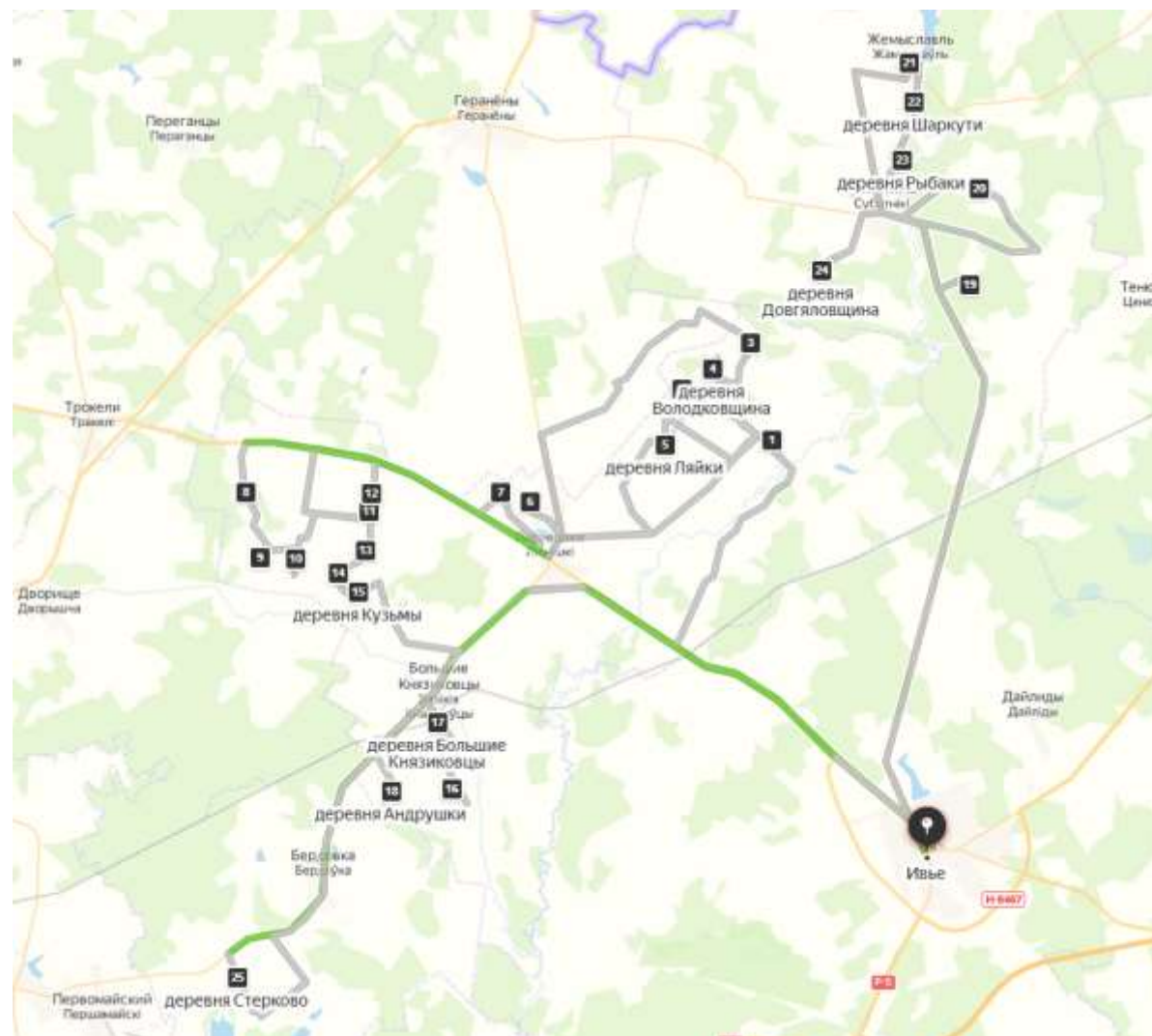
Рисунок 9 – Маршрутный график сбора и удаления ТКО машина 1 2я и 4я сб.
