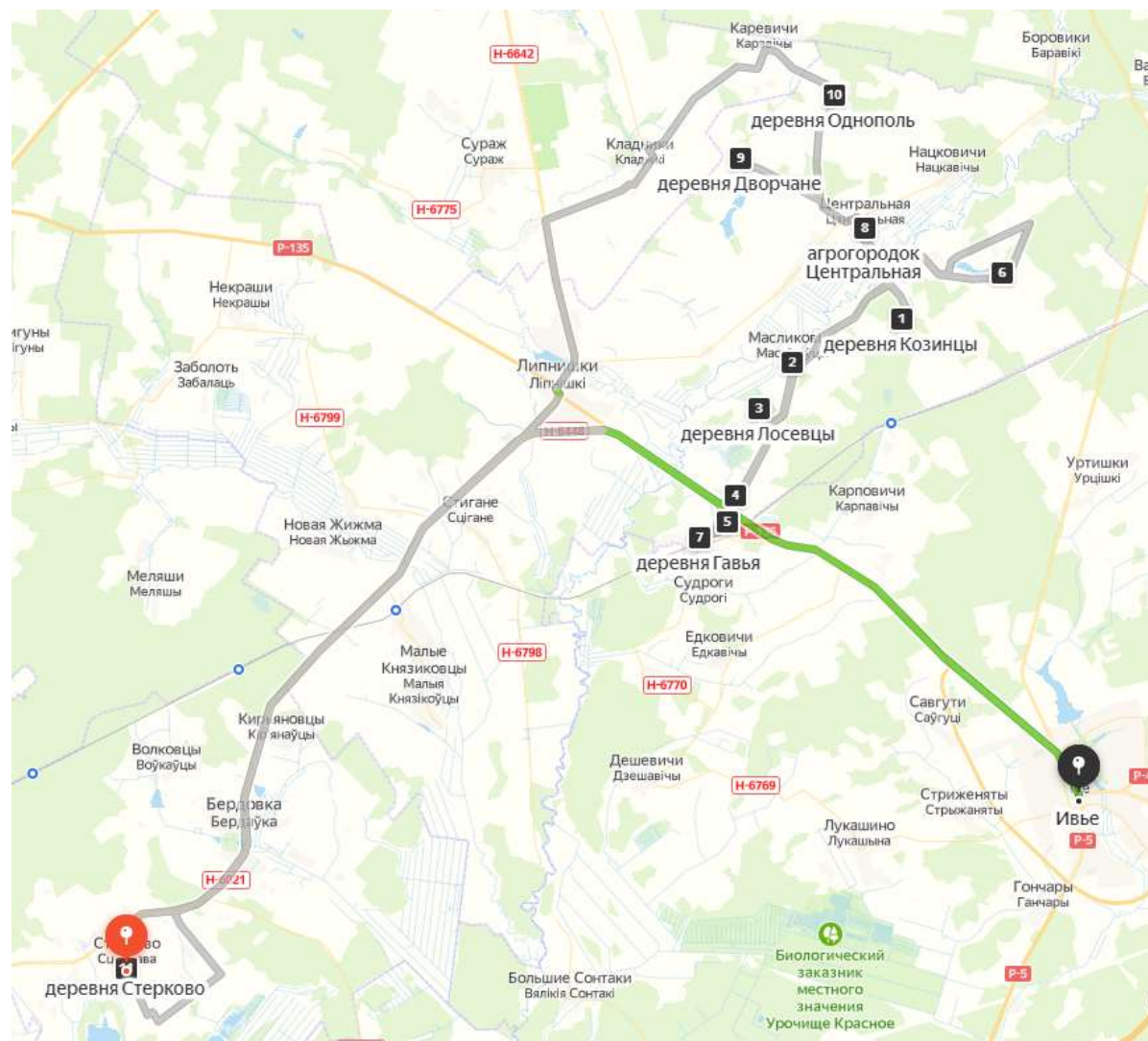
Рисунок 36 – Маршрутный график сбора и удаления ВМР машина 2 4я ср. Рейс 2
