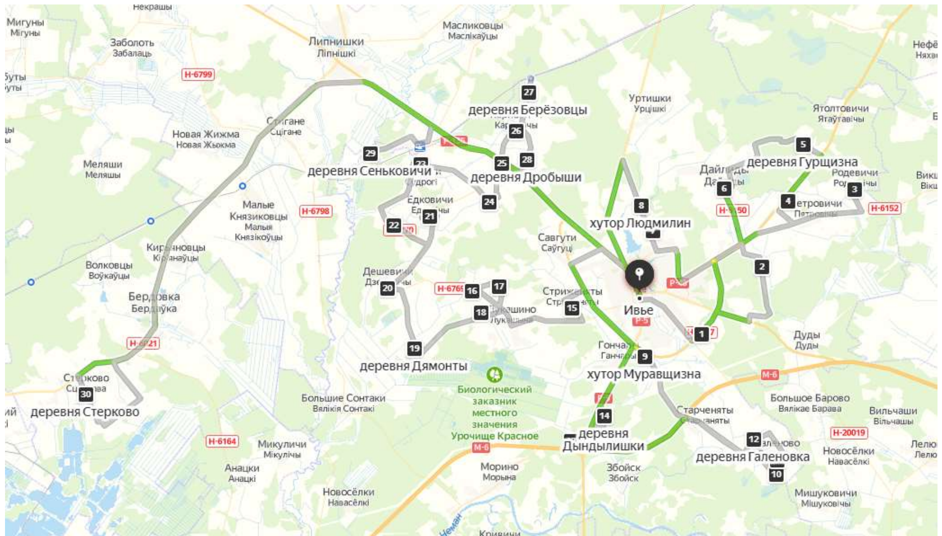
Рисунок 5 – Маршрутный график сбора и удаления ТКО машина 1 2й и 4й пп.
