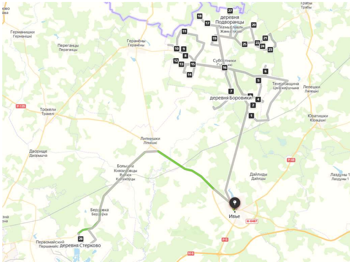
Рисунок 10 – Маршрутный график сбора и удаления ТКО машина 1 2с и 4с вс.
