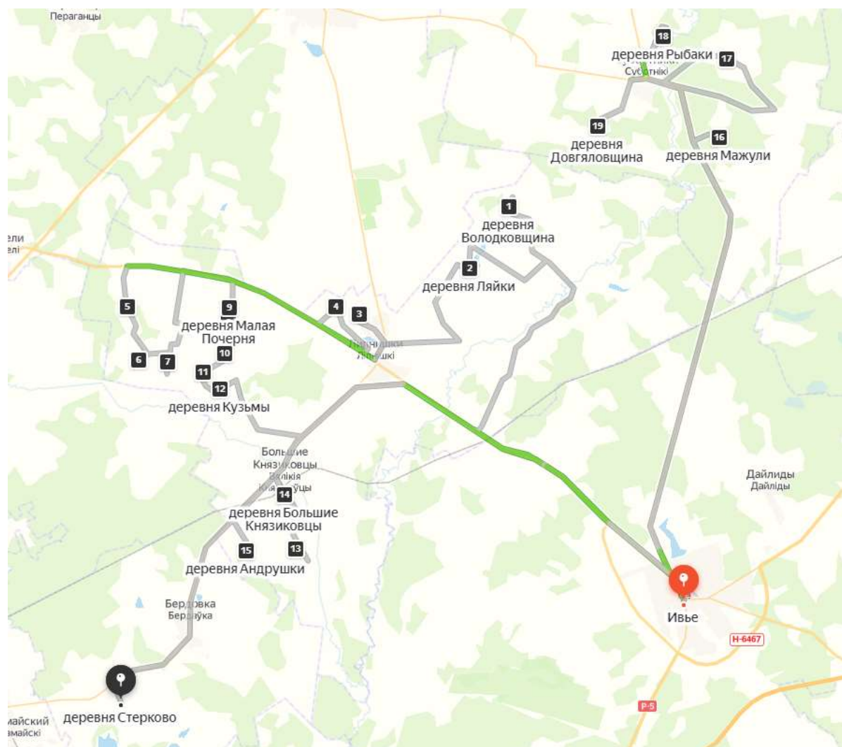
Рисунок 37 – Маршрутный график сбора и удаления ВМР машина 2 4й чт. Рейс 1
