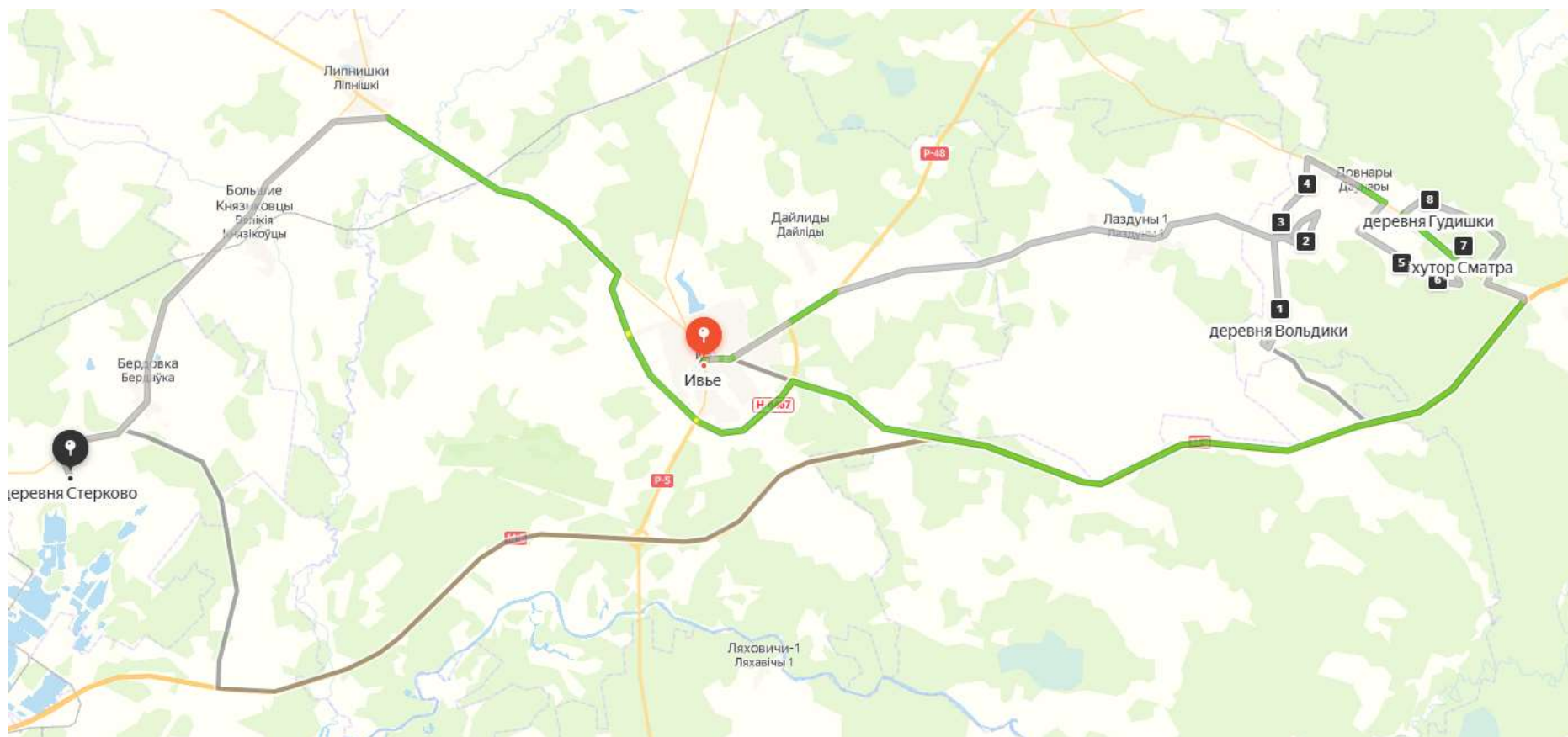
Рисунок 15 – Маршрутный график сбора и удаления ВМР машина 2 2й пн. Рейс 1,2
